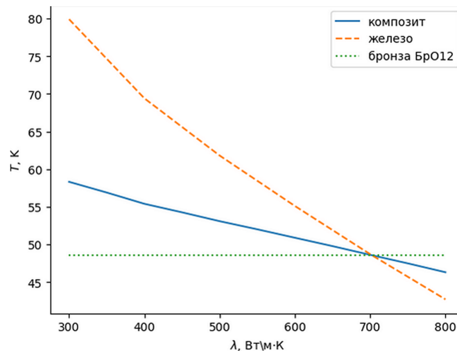
Рис. 1. Зависимость коэффициента теплопроводности композита БрО12-Fe от температуры
